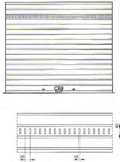
Feritoie di aerazione per profili CM 10 - CM 14 - CM 10 W
