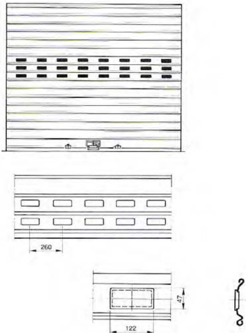
Finestratura (122 x 47 mm. passo 260 mm.) per profili CM 10 - CM 14 - CM 10 D
