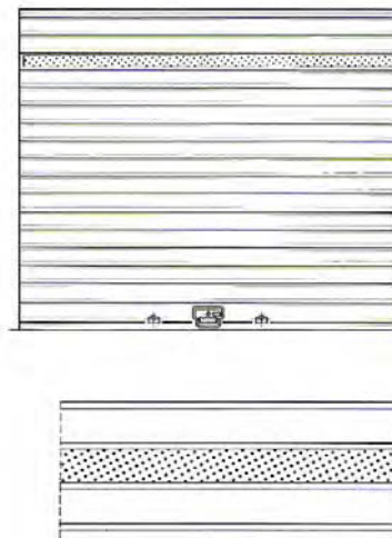
Elemento microforato CM 10 - CM 10 S - CM 7
