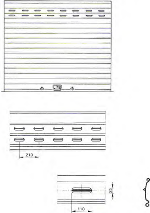
Feritoie di aerazione per profili CM 10 - CM 14 - CM 7
